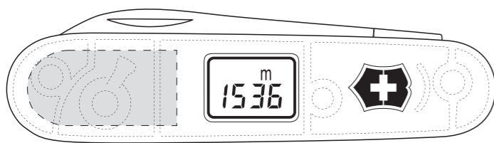
Frente translúcida siempre con emblema, longitud 91 mm, Traveller y Voyager
